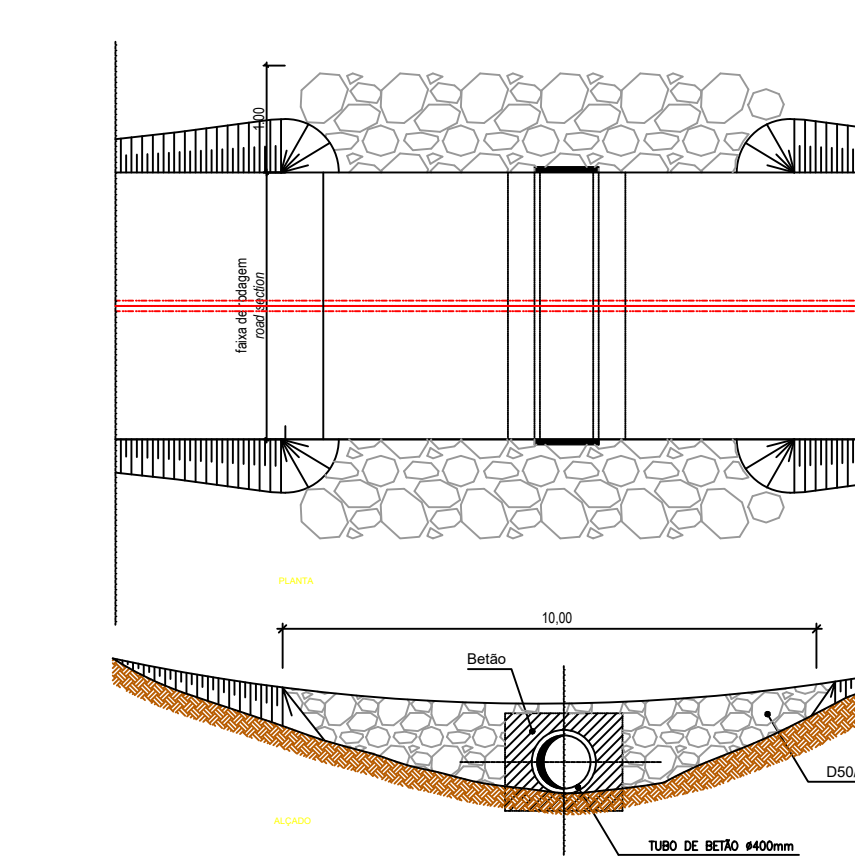
PASSAGEM NÃO GALGÁVEL COM MANILHAS Ø400 - TIPO 3 Pipe River Passage Ø400 - Type 3
