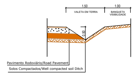
VALETA DE PLATAFORMA TIPO 1 ROAD DITCH TYPE 1
