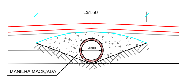
CONTINUIDADE DE VALETAS SOB SERVENTIAS - TIPO 4 COM MANILHAS (300mm) E REVESTIMENTO SUPERIOR EM BETÃO ACCESS ROAD DITCH PASSAGE IN CONCRETE - TYPE 4
